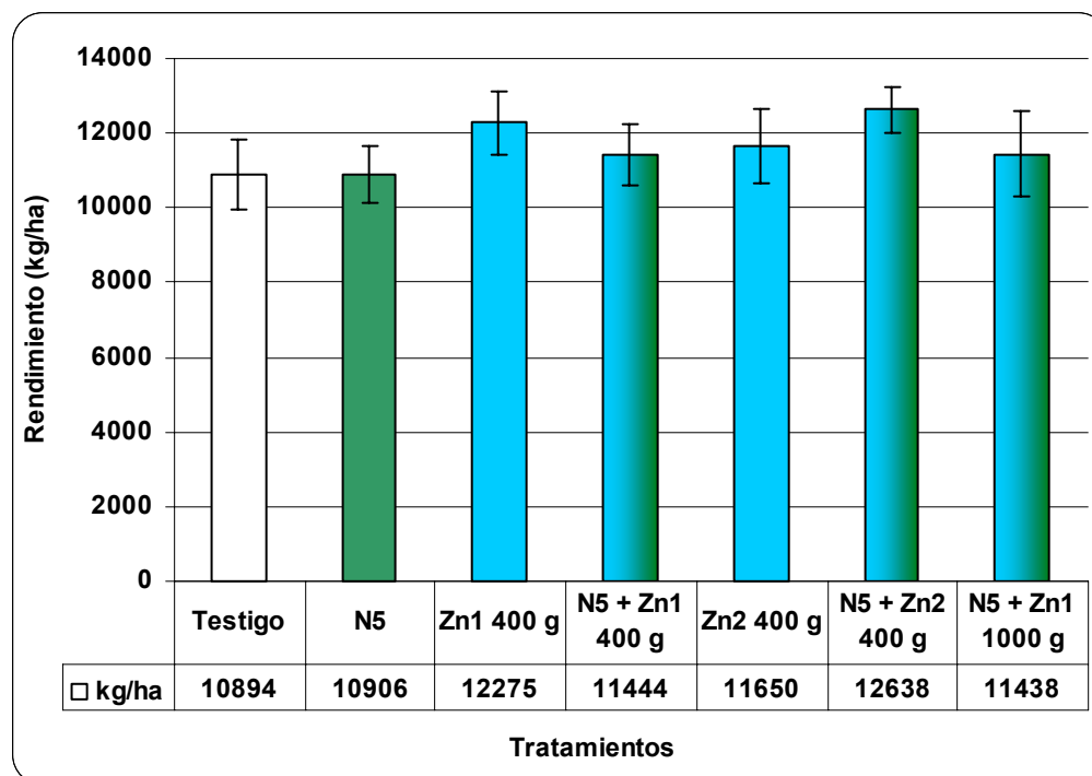
Figura 5: Rendimiento (kg ha -1 ) como resultado de la aplicación de nitrógeno y zinc foliar en maíz.. Columna blanca representa al testigo, columna verde tratamiento con nitrógeno, columnas celestes tratamientos con zinc, columnas bicolors aplicaciones conjuntas de nitrógeno y zinc. Las barras verticales indican la desviación Standard de la media. Pergamino, Campaña 2007/08.
