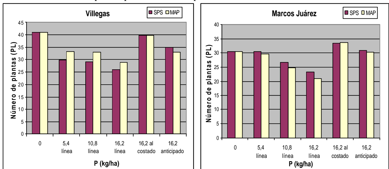
FIGURA 1: Número de plantas por Ha en cada experiencia
