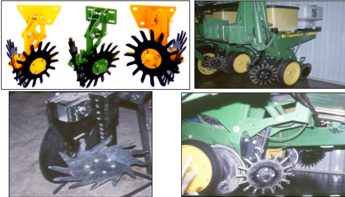
Figs. 4,5,6 y7: diferentes tipos de barredores de rastreo articulados, fijos y su colocación en el cuerpo de siembra.
