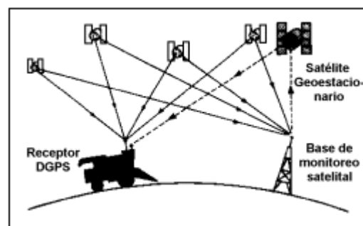
Fig. 2: Esquema de la señal satelital
