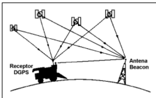
Fig. 1: Esquema de señal de Beacon
