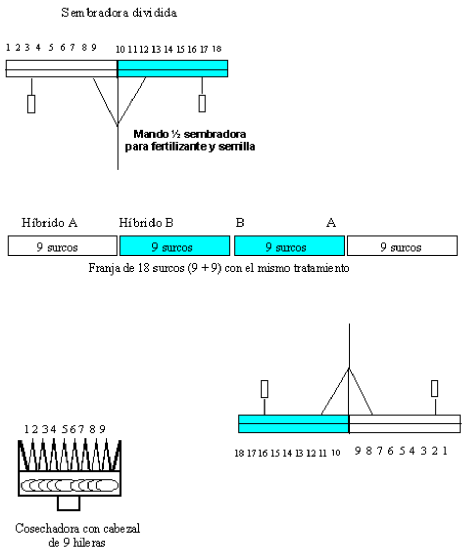
Fig. 13: Esquema de metodología de trabajo de franjas apareadas para la posterior confección de mapas de diferencias.
