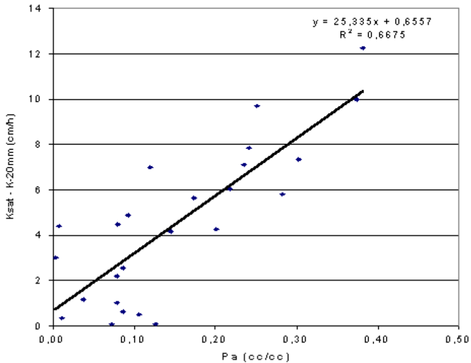
Graf.: 4. Relación entre la conductividad hidráulica de los macroporos medida, y la porosidad de aireación (Pa) en suelos Argiudoles Típicos de la Pampa Ondulada
