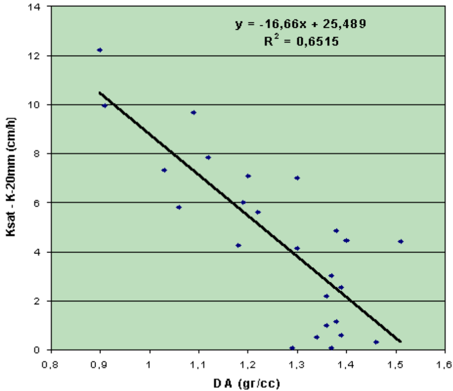
Graf.: 3. Efecto del aumento de la DA sobre el funcionamiento de la macroporosidad en suelos Argiúdoles Típicos de la Pampa Ondulada
