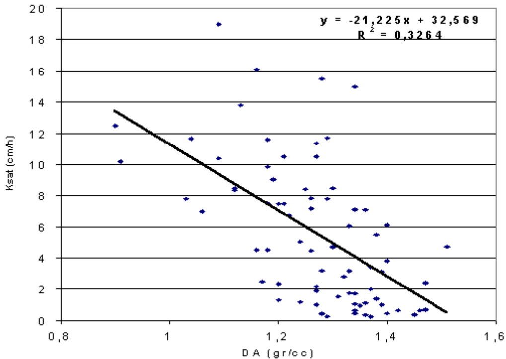
Graf.: 1. Variación de la Ksat con el aumento de la DA en suelos Argiúdoles Típicos de la Pampa Ondulada
