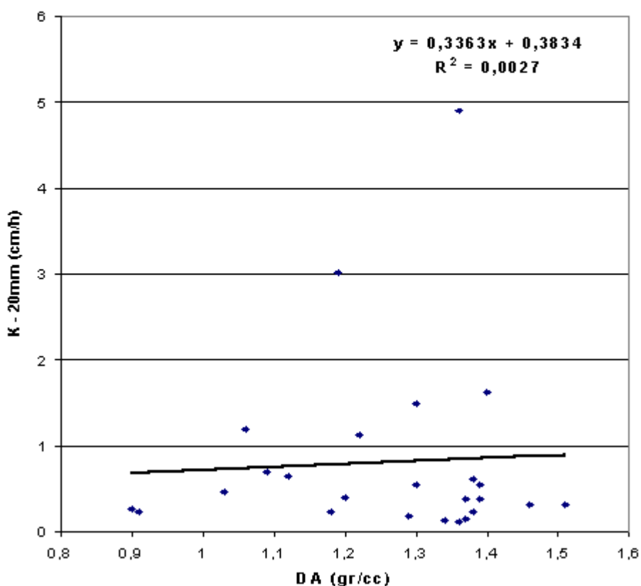
Graf.: 2. Variación de la K no saturada (-20mm) con el aumento de la DA en suelos Argiúdoles Típicos de la Pampa Ondulada
