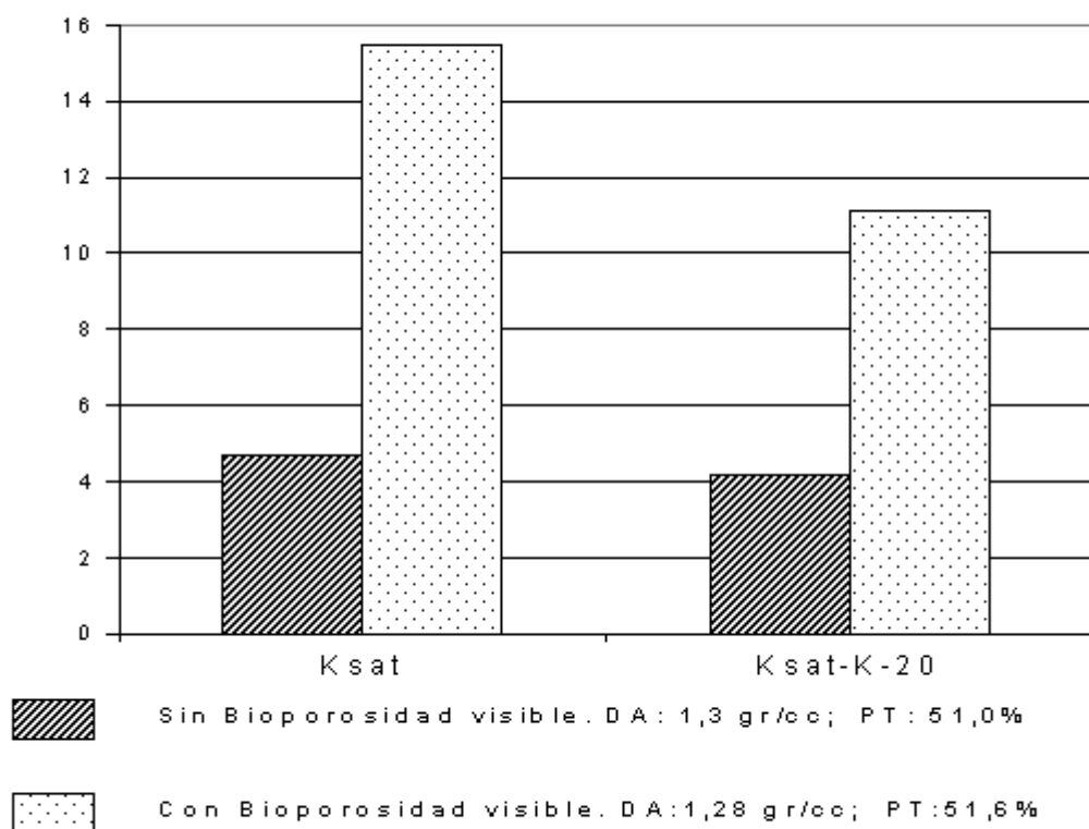
Graf.: 7. Variación de la Ksat por efecto de la Bioporosidad en suelos Argiúdoles Típicos de la Pampa Ondulada
