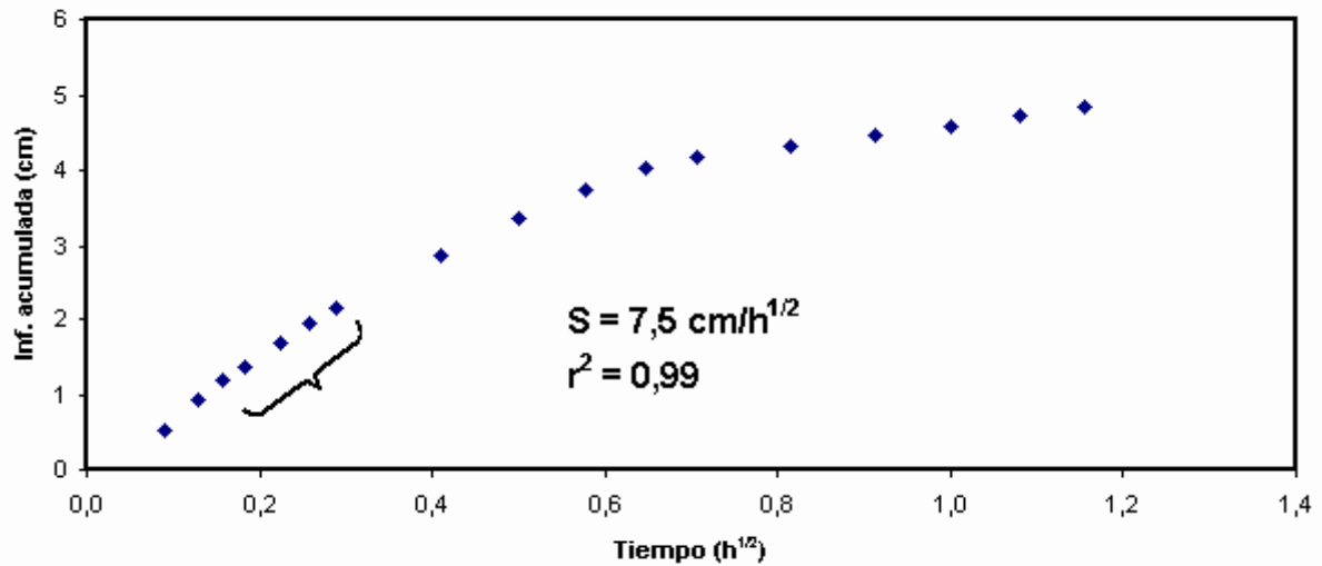
Graf. 2: Sortividad
