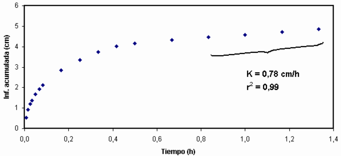
Graf. 3: Flujo Estacionario
