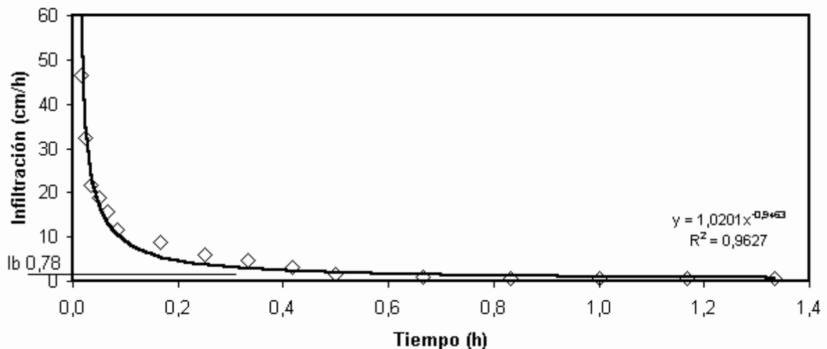
Graf. 1: Tasa de Infiltración
