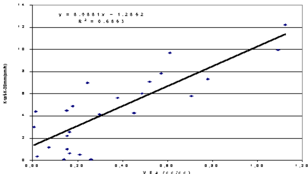
Graf.: 5. Relación entre la conductividad hidráulica de los macroporos y el volumen específico de aireación en suelos Argiúdoles Típicos de la Pampa Ondulada
