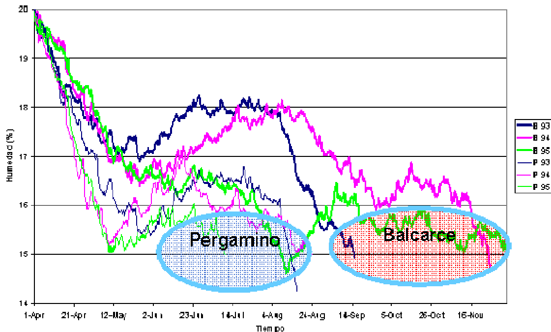
Figura 3. Contenido de humedad promedio del maíz durante el secado en silo con aire natural para las localidades de Pergamino (líneas finas) y Balcarce (líneas gruesas) para los años 1993 a 1995. Humedad inicial: 20%; humedad final: 15%; fecha de inicio: 1 de abril; caudal de aire: 1m 3 min-1t-1.
