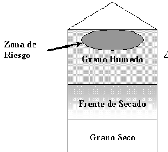
Figura 1. Distribución de la humedad en la masa de granos durante el secado en silo con aire natural o baja temperatura y conformación de la zona de riesgo de descomposición de granos en la parte superior y central del granel.
