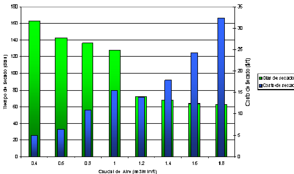
Figura 2. Tiempo y costo de secado para caudales de aire entre 0.4 y 1.8 m 3 min -1 t -1 . Simulación hecha con datos climáticos de Pergamino. Los costos de secado deben tomarse de manera indicativa para comparar diferentes caudales de aire.
