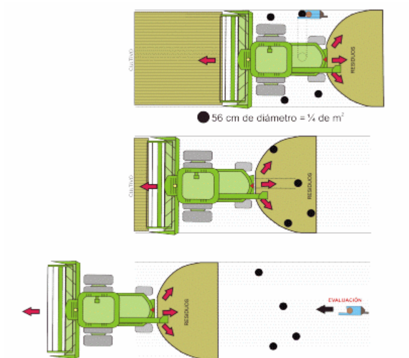
Figura 2: Disposición de los aros ciegos para muestreo de pérdidas de granos por cabezal y cola.
