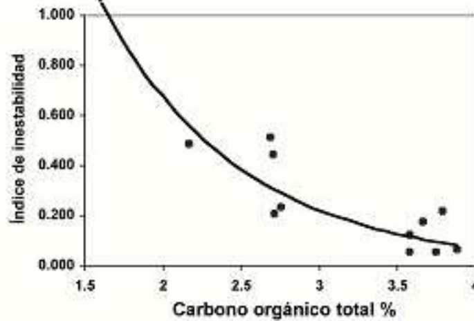
Fig. 7. Relación entre el Is y el COT del suelo en la Serie Santiago.
