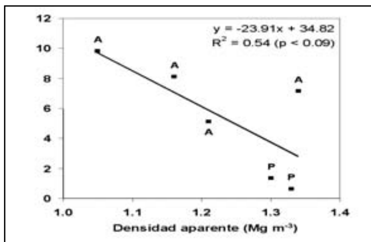
Fig. 1: Densidad aparente máxima según contenidos de materia orgánica o de arena en 5 molisoles de la región de la pampa arenosa según métodos de estimación. P = suelos bajo pasturas, A = suelos en agricultura.
