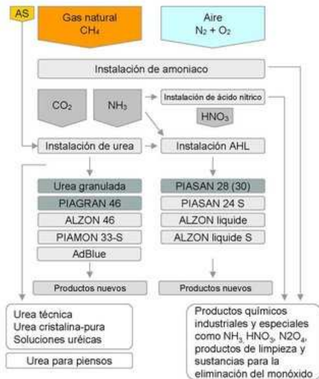
Proceso de elaboración de abonos minerales
